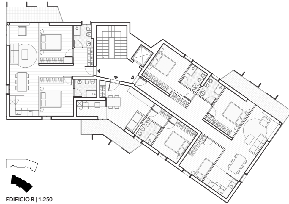
EDIFICIO B | 1:250
