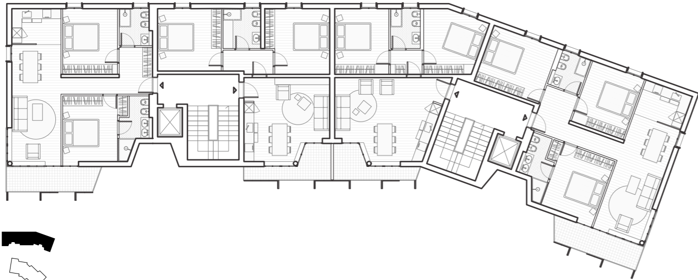
EDIFICIO A | 1:250
