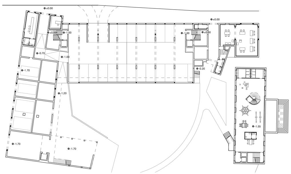
Pianta quota ± 0.00, sc. 1:500
