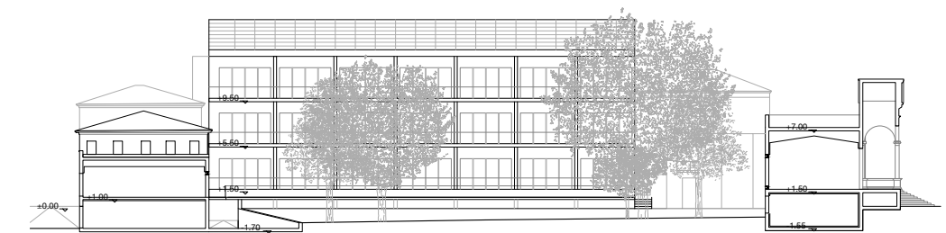
Sezione DD, sc. 1:500
