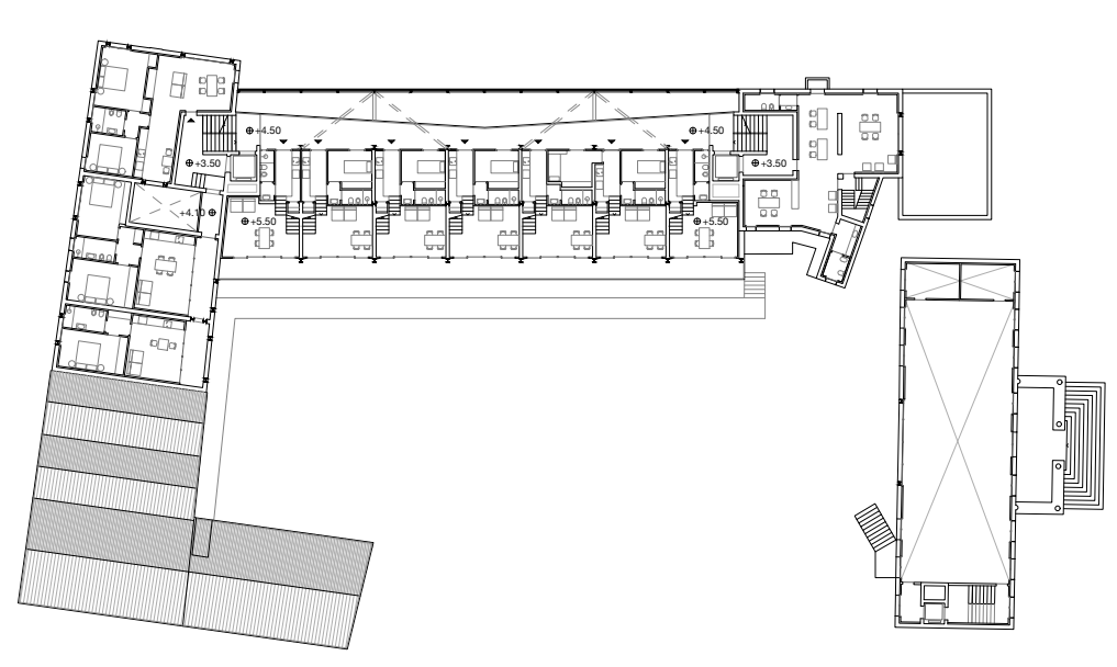
Pianta quota +4.50, sc. 1:500
